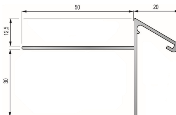
Modèle encastré 12,5 mm
