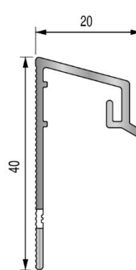
Modèle rapporté de 3,0 m (permettant l'utilisation des accessoires)
